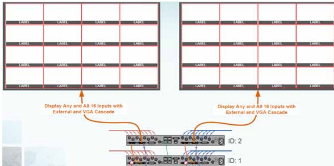
Rainier 3G 2台カスケードでのシステム例
